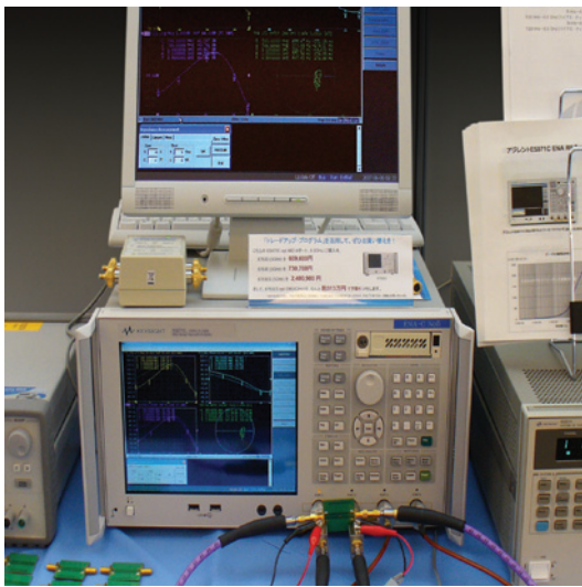
直流偏置的测量设置
