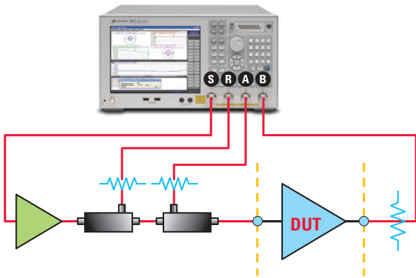
使用外部测试设置模式进行大功率测量
