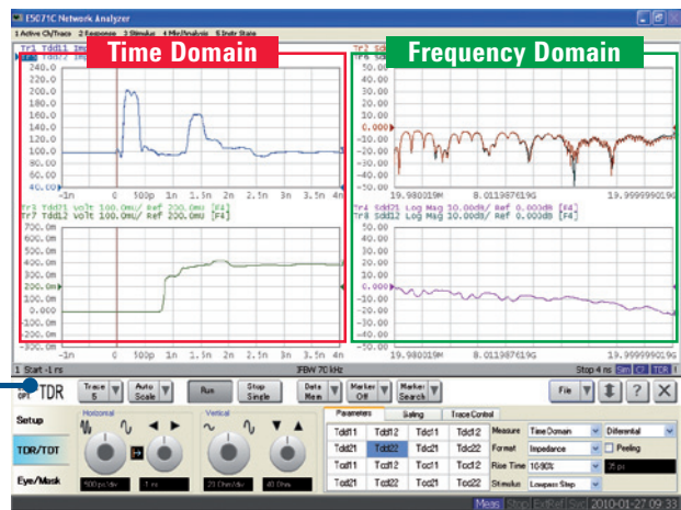
可同时进行时域分析和频域分析
